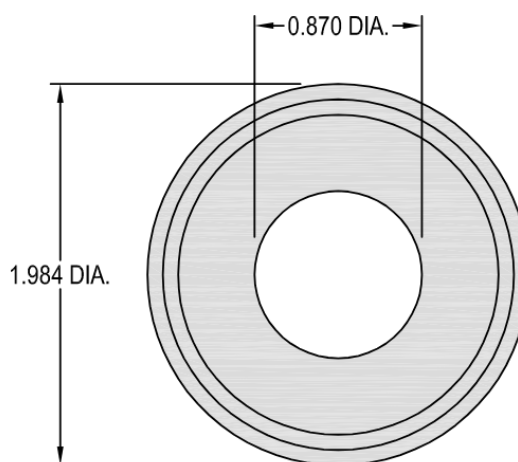
1" T.C.
